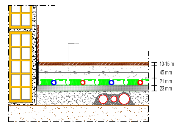
SEZIONE PANNELLO PREFORMATO PIANI INTERMI
