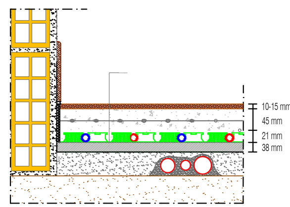
SEZIONE PANNELLO PREFORMATO PIANO TERRA
