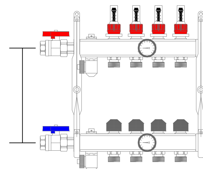
ESEMPIO COLLETTORE DI DISTRIBUZIONE
